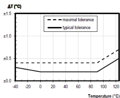
図 内蔵センサーの基準温度誤差
