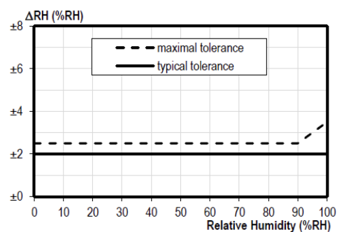
図 内蔵センサーの基準湿度誤差
